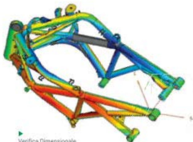
Verifica Dimensionale Telaio Moto
